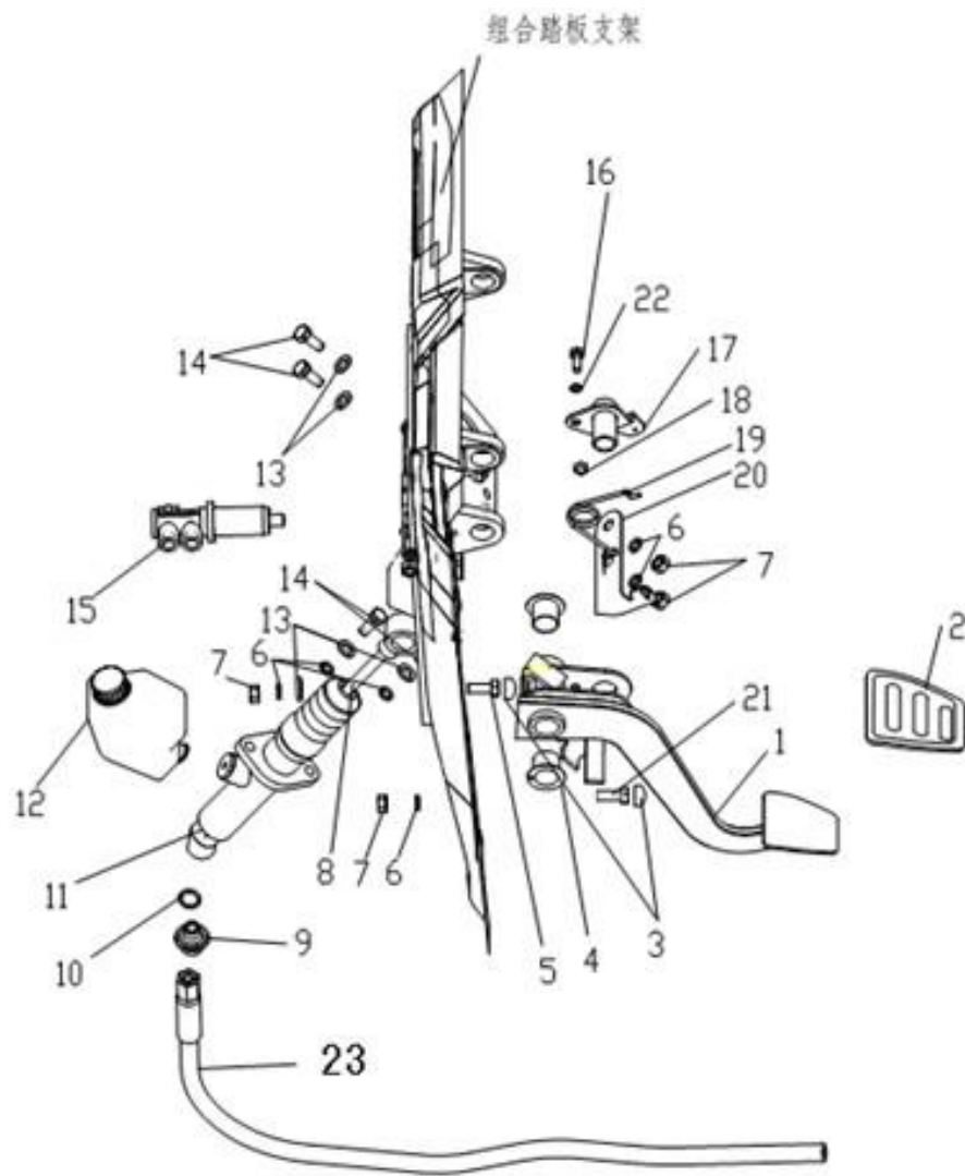
驾驶室部分
